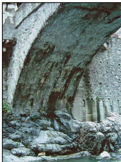
Volta del ponte con i segni dell'ampliamento avvenuto nel 1606 (a sinistra) e Chiesa di San Carlo ai Tetti, dei primi decenni del XVII secolo (a destra).
